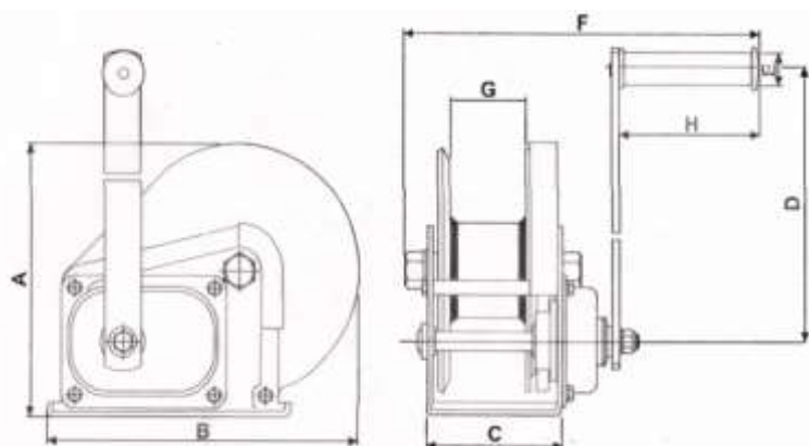
Рис. 1 - Габаритные размеры лебедки ЛБ (ВНВ)
